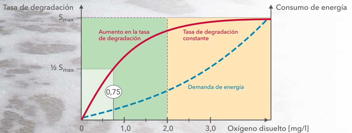
Dependencia de la degradación \text{NH}_4\text{-N} de la concentración de oxígeno.
