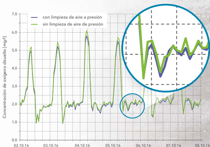
Comparación de dos sensores FDO® con y sin limpieza de aire a presión
